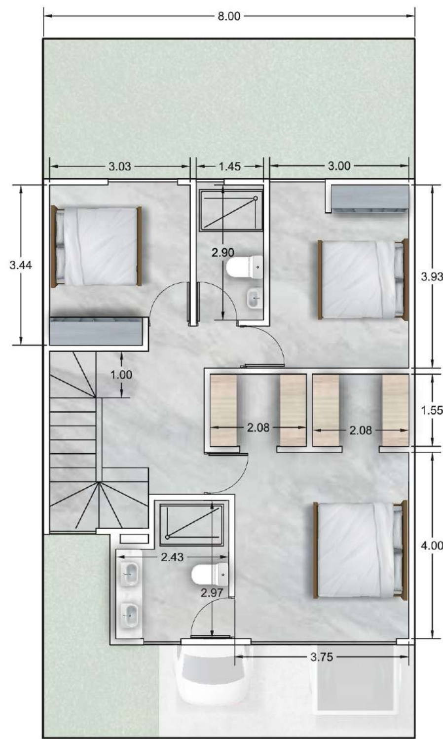
SEGUNDA PLANTA
